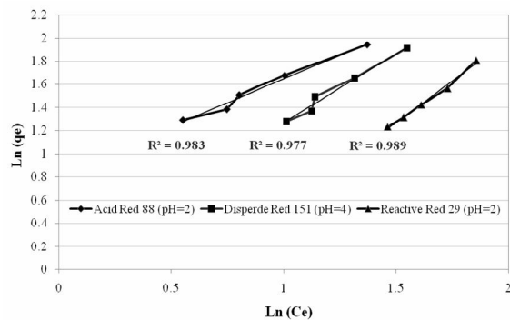
شکل ۱- نمودارهای ایزوترم جذب فروندلیچ برای هر رنگینه
